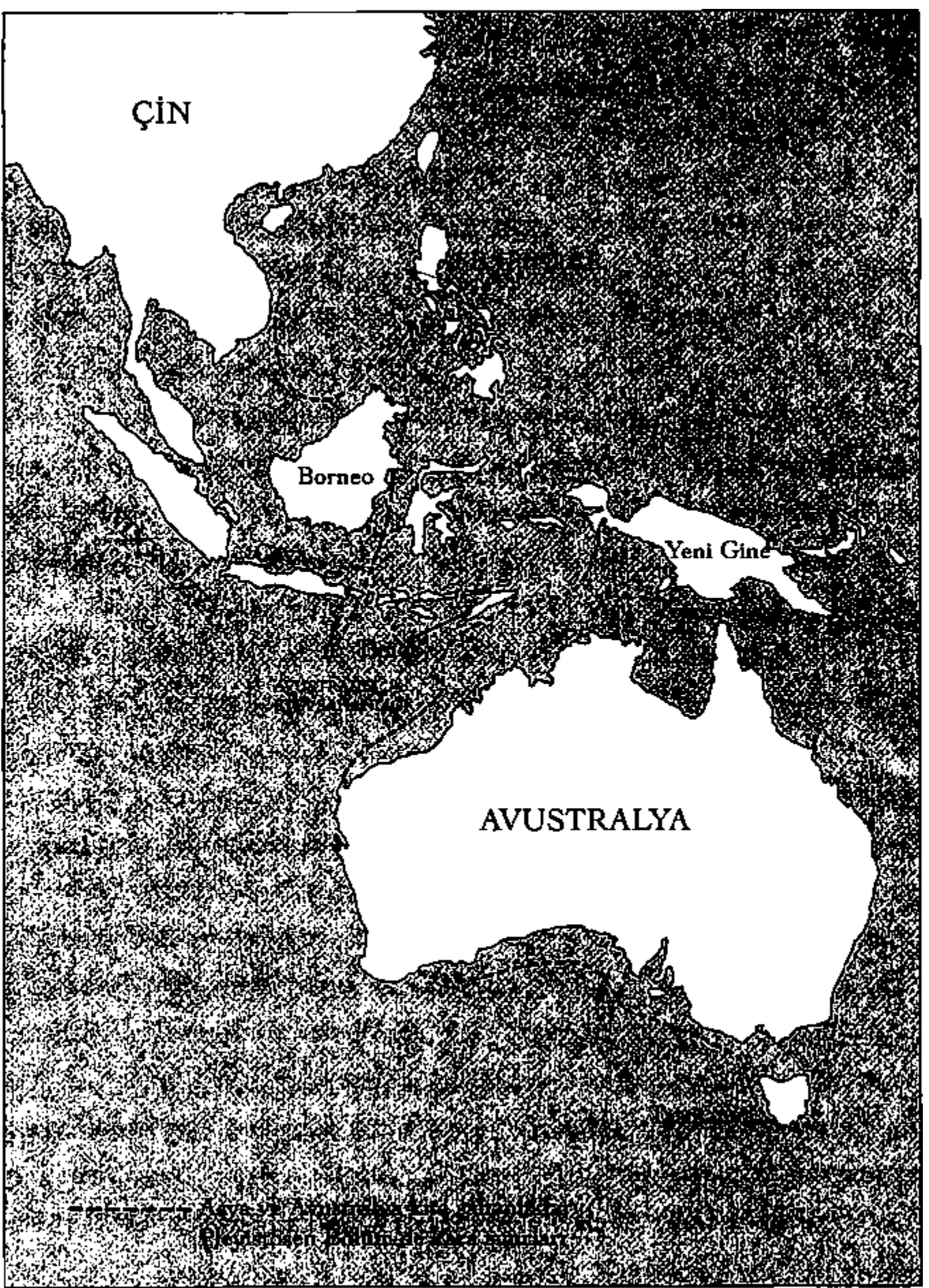
Şekil 15.1. Güneydoğu Asya'dan Avustralya ve Yeni Gine'ye kadar bölge haritası. Kesiksiz çizgiler bugünkü kıyıları
