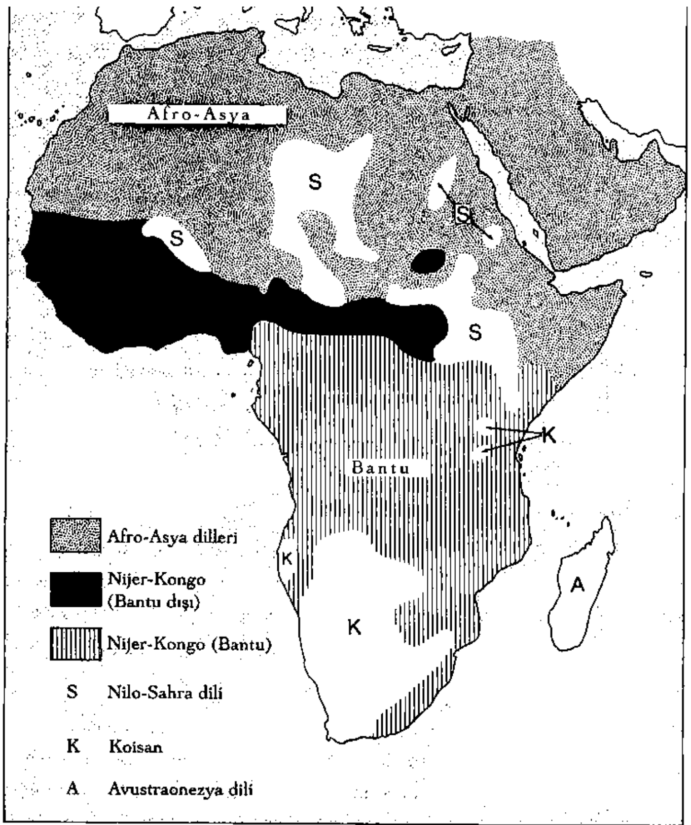
Şekil 19.2. Afrika'daki dil aileleri.
