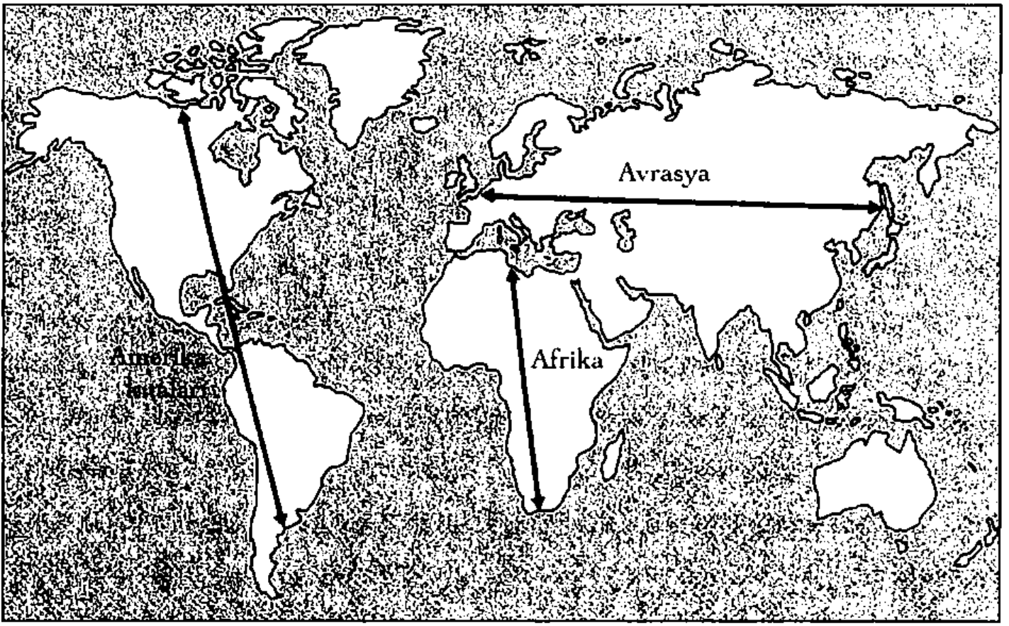
Şekil 10.1. Kıtaların ana eksenleri.
