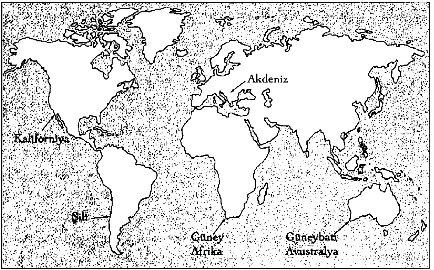
Şekil 8.2. Dünyadaki Akdeniz İklim Kuşakları.
